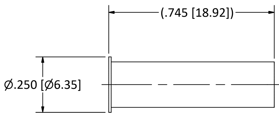
VIEW1 SCALE 4 : 1
